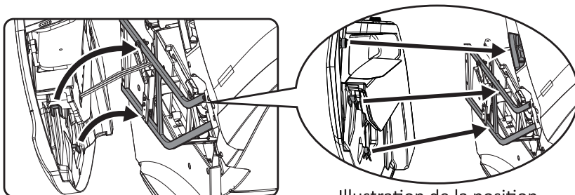
Illustration de la position d'accostage du crochet
